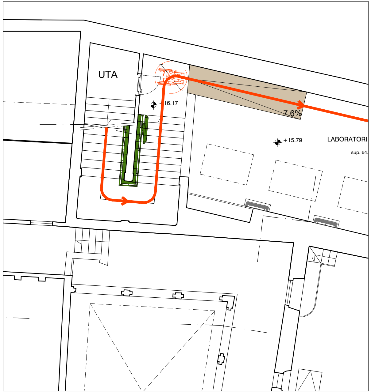
PIANO TERZO
