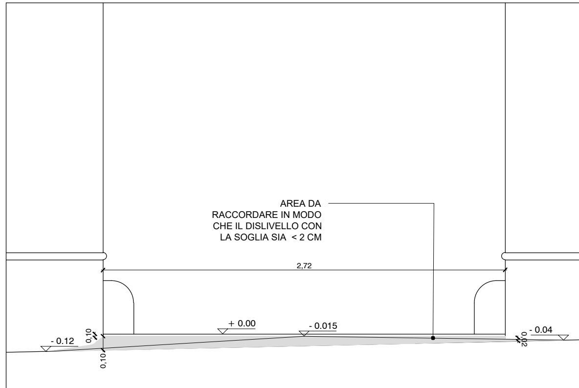
PROSPETTO - 1:25
