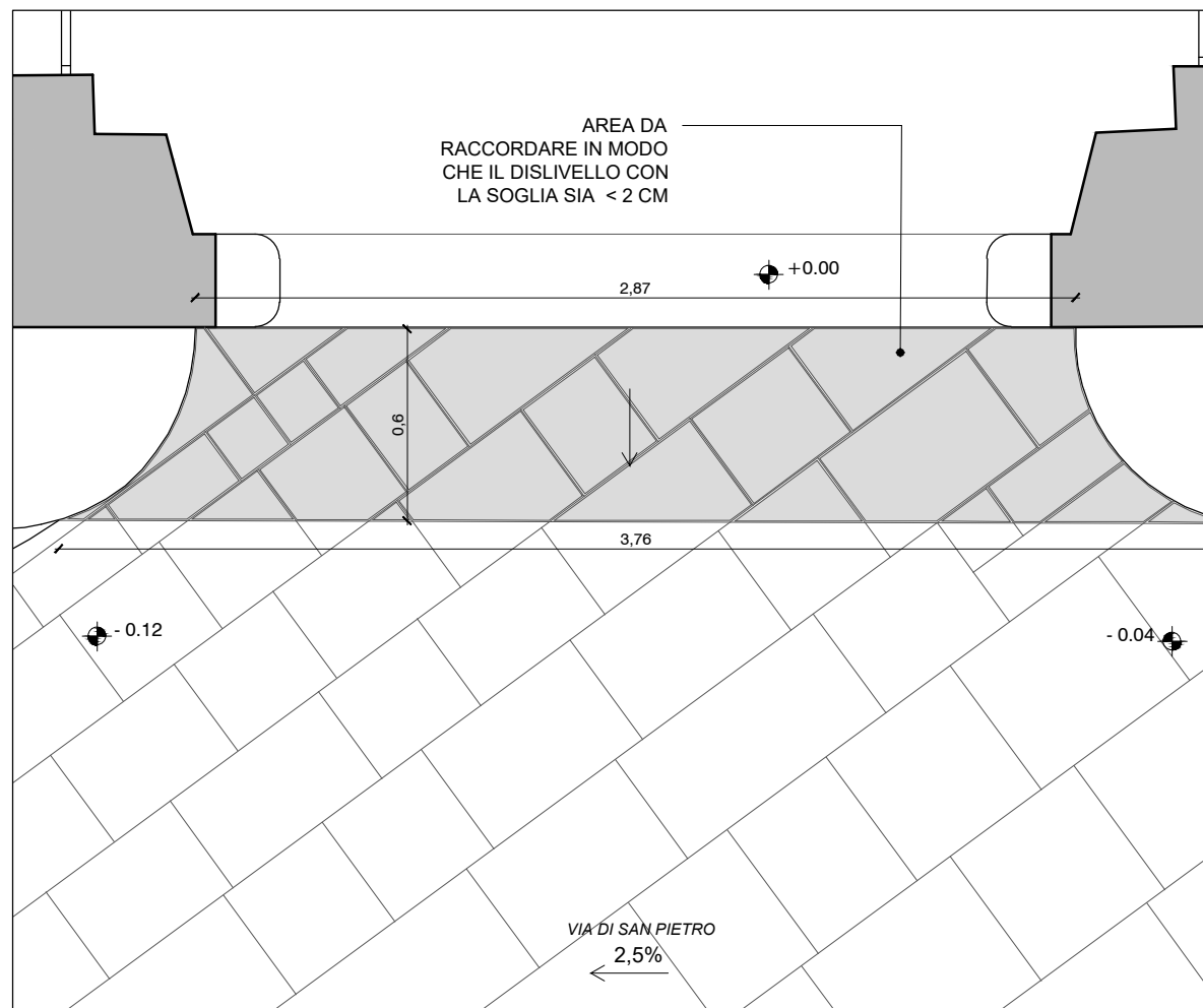
PIANTA - 1:25
